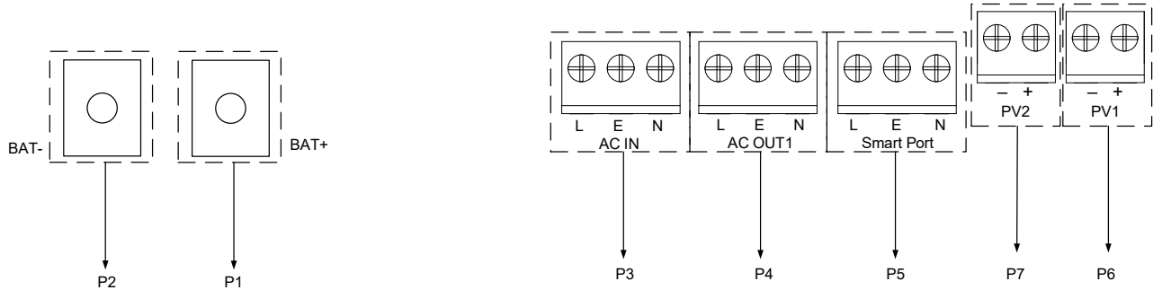
MPPT Module Ver V1.0
