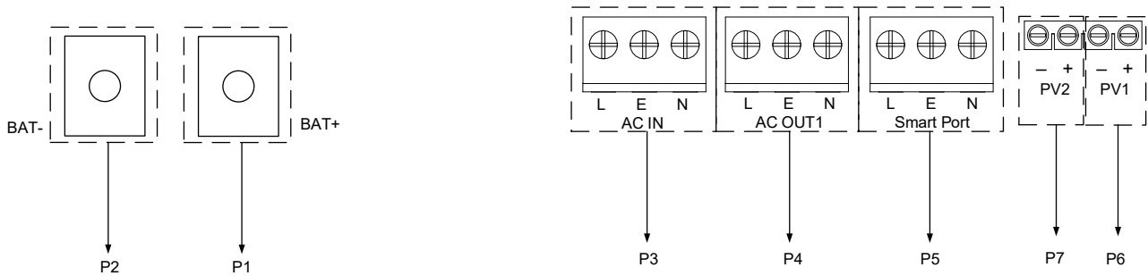
MPPT Module Ver V2.0 5KVA-S, 6KVA-S, 8KVA-S, 8KVA-S Pro Power Port
